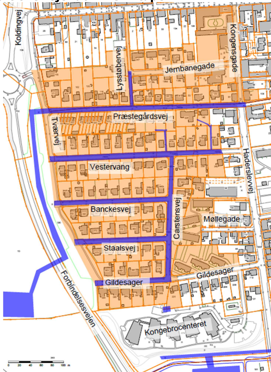
Figur 1 Orange - Ejendomme berørt af Etape 4. Blå hvor vi etablerer nye kloakledninger ved opgravning eller ved boring.
